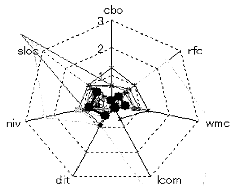
図 10 その他のクラス (サンプル数 39)
