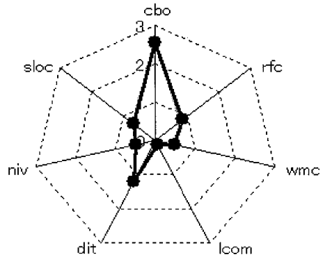
図 8 CWinApp 派生クラス (サンプル数 17)
